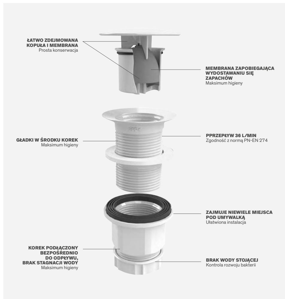
Przekrój 621W: spust bezwodny Nr DELABIE: Przekrój3D_621W
